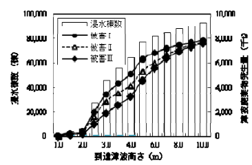
到達津波高さと津波廃棄物発生量の関係 (徳島市域)
