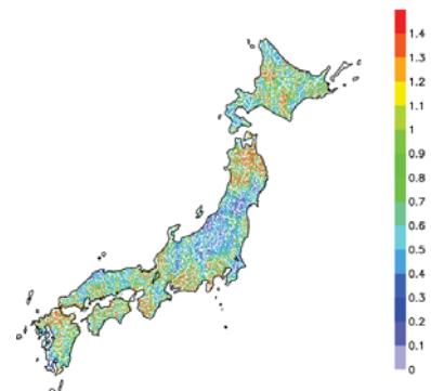
現在気候に対する21世紀末気候との比率(気象庁気象研究所の)超高分解度 全球大気モデル(Mizuta et al., 2012)を用いて計算した、再現期間100年の年最 大流量の変化率(立川ら, 2011; 文部科学省, 2012)。
