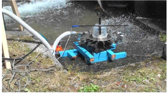
小水力発電機の開発
