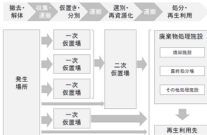
図 2-5-5 全体的な災害廃棄物処理の流れ
