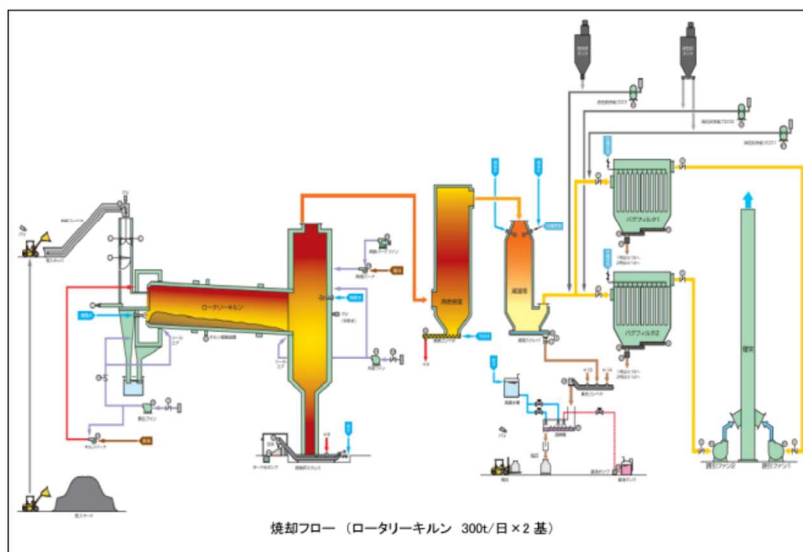
図 2-5-2 ロータリーキルン炉の処理フロー
