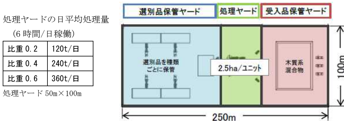
図 2-10-6 木質系混合物処理施設（移動式）の基本ユニット
