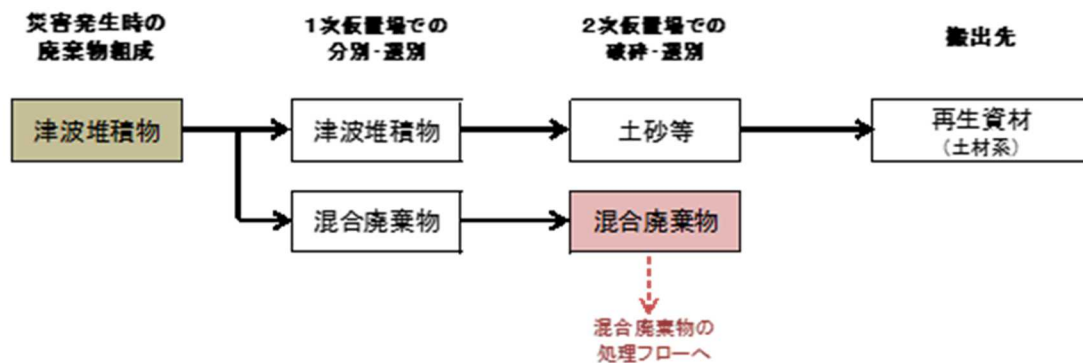
図 2-5-9 津波堆積物処理フロー
