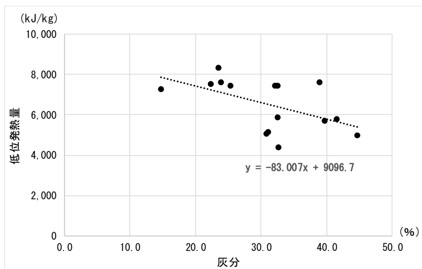
図 2-6-2 灰分と低位発熱量
