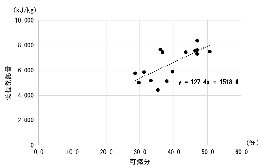
図 2-6-1 可燃分と低位発熱量
