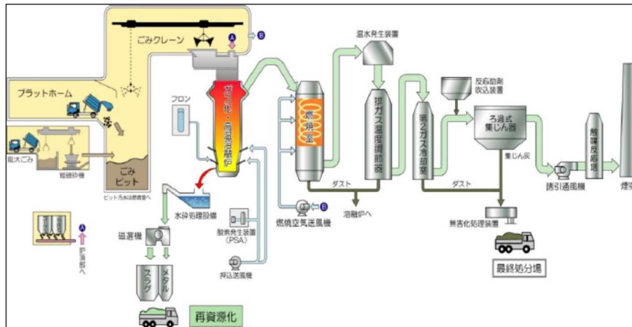
図 2-5-3 シャフト炉の処理フロー
