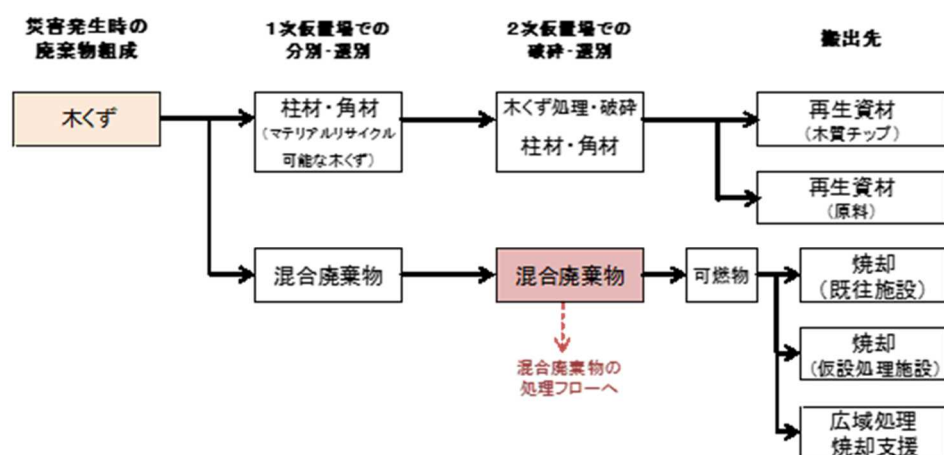
図 2-5-6 木くず処理フロー
