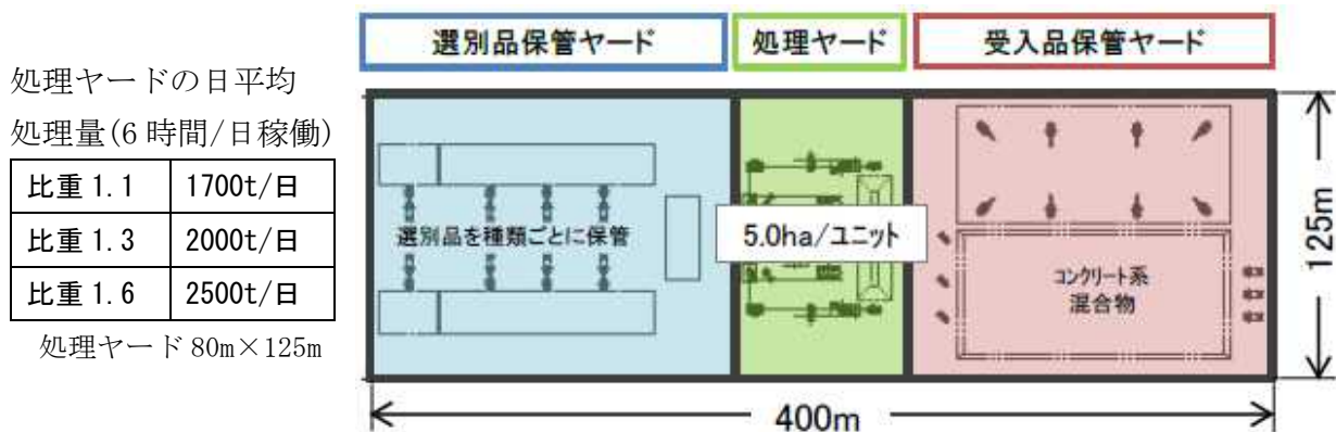
図 2-10-5 コンクリート系混合物処理施設（固定式）の基本ユニット
