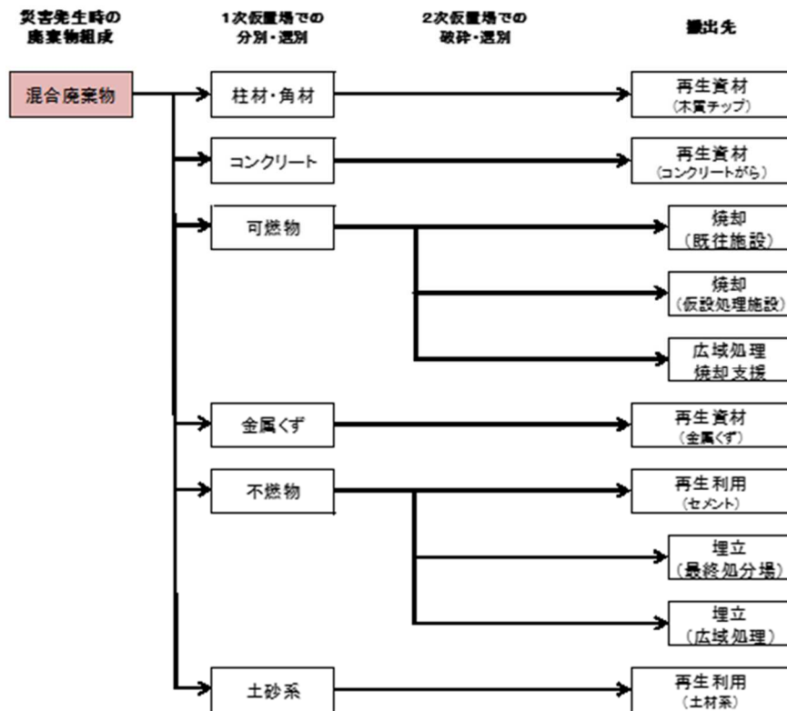
図 2-5-11 発生した混合廃棄物の全体的な処理フローの例
