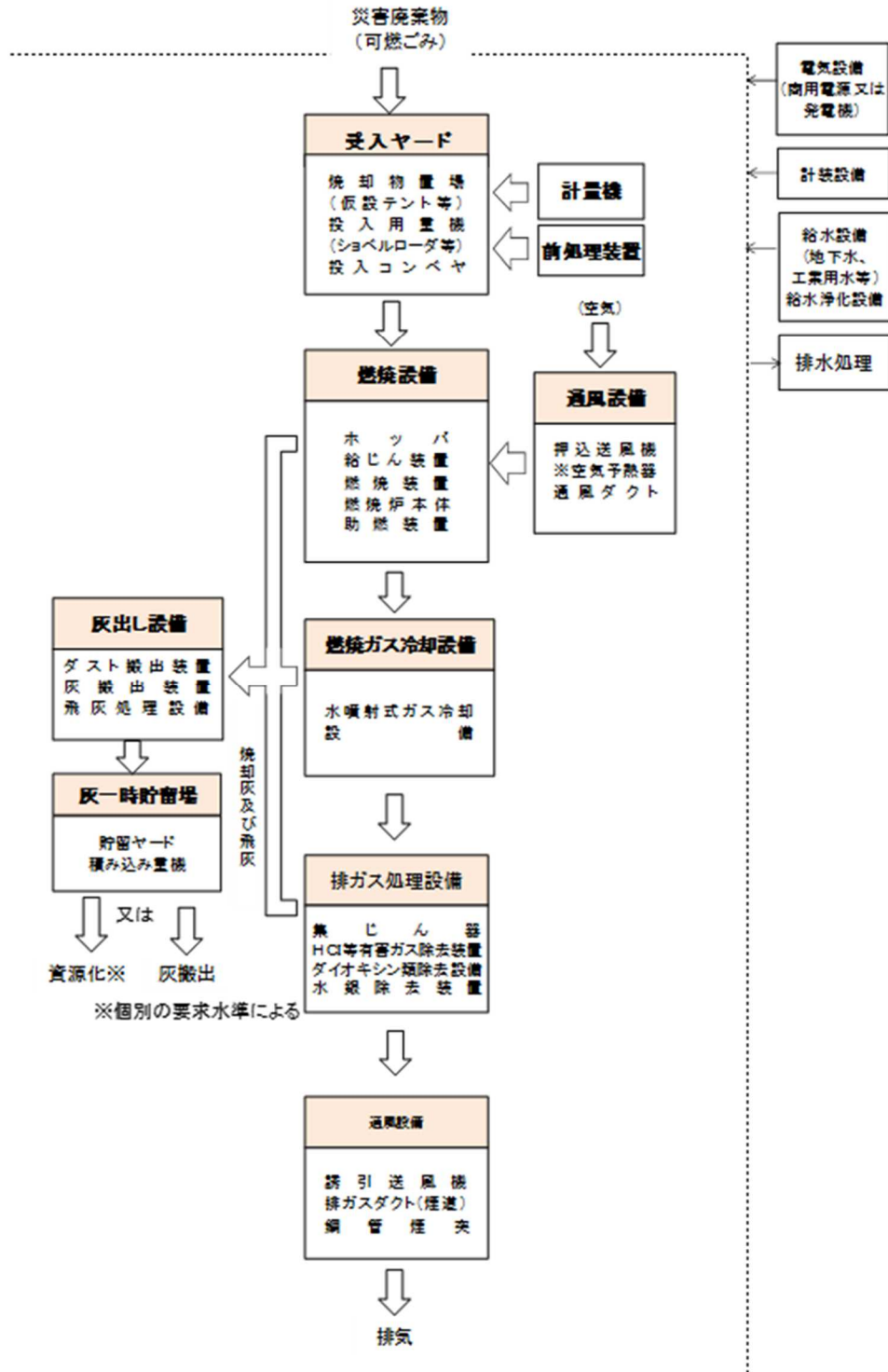
図 2-5-4 仮設焼却処理施設の標準フロー
