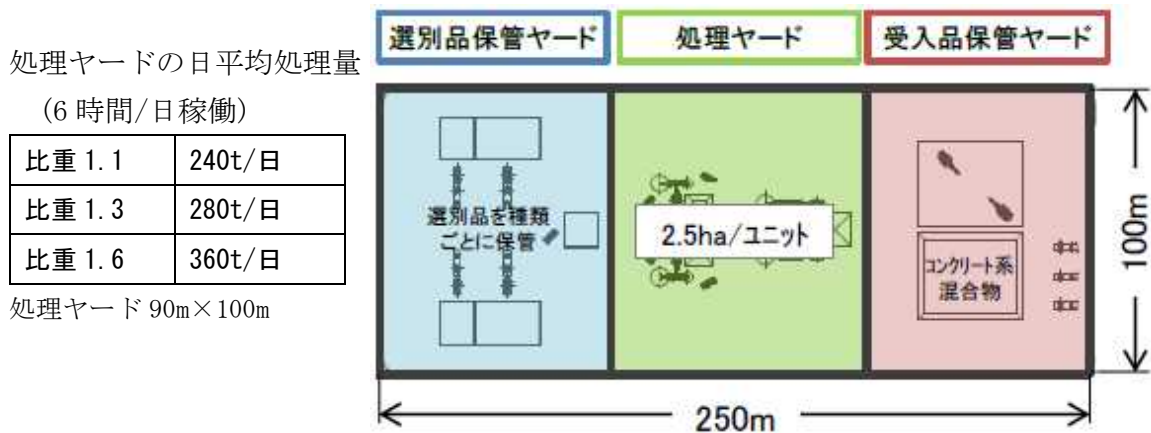
図 2-10-4 コンクリート系混合物処理施設（移動式）の基本ユニット
