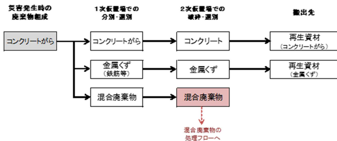
図 2-5-7 コンクリートがら処理フロー
