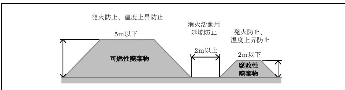
図 2-12-1 可燃性廃棄物の管理
