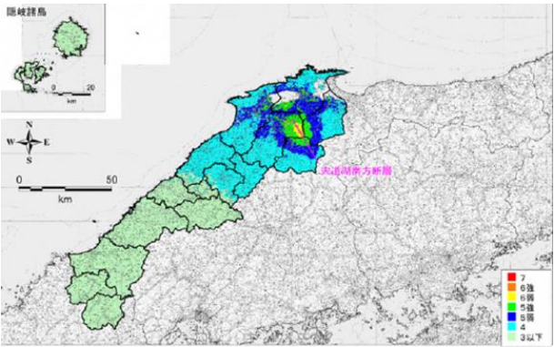
図 3.1 宍道湖南方断層の地震における震度分布
