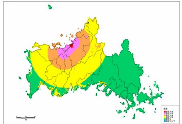
図 5.1 萩北断層の地震における震度分布
