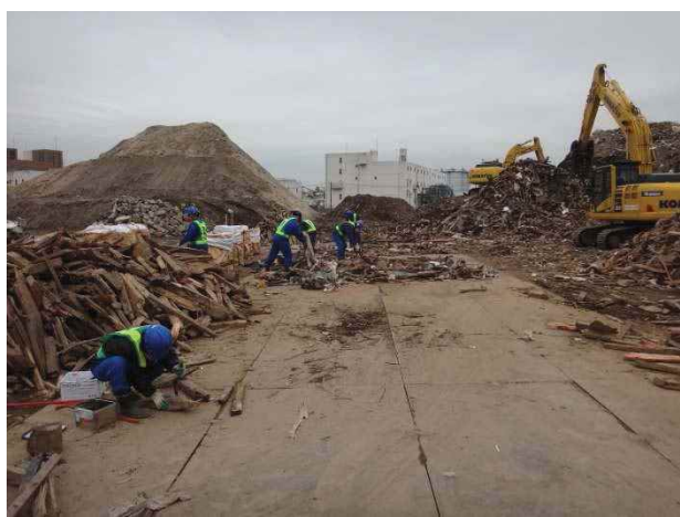
7 下水道局西部水資源再生センター用地 【H27. 2.26 作業風景】
